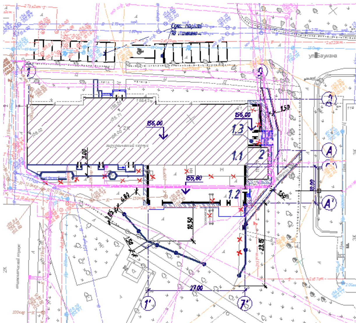
Рисунок 8 – Схема объекта проектирования
